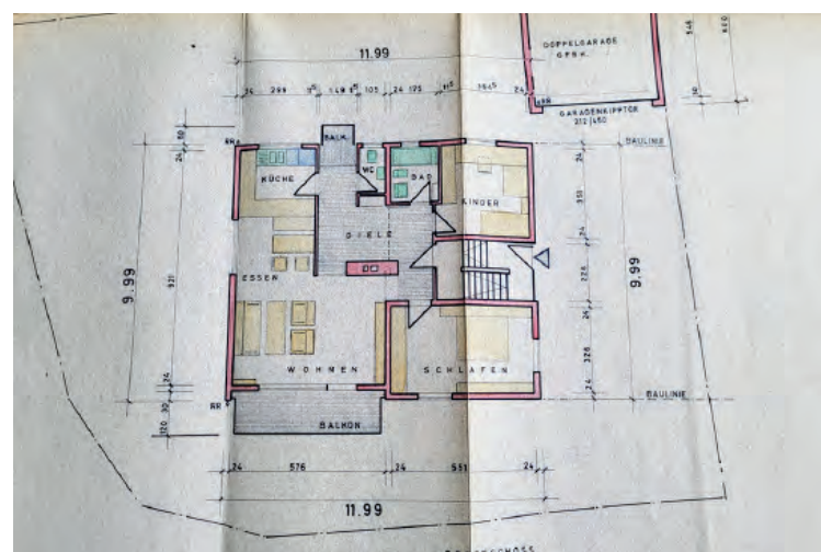
Bauplan-Skizze Erdgeschoss
