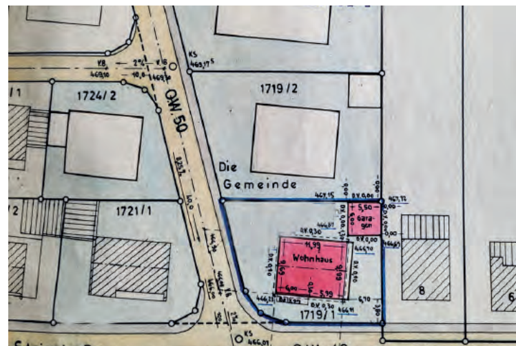
Lageplan
